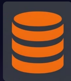
SQL Database
